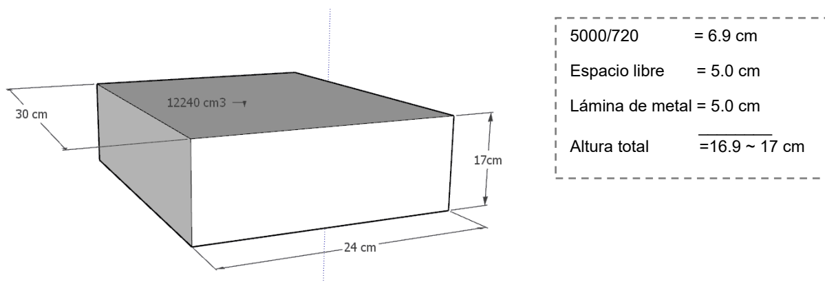
Figura E.6 - Ejemplo de las dimensiones de la superficie de la olla de BoPET para cada una de las dos ollas en contacto con la plancha de 40 cm por 60 cm
