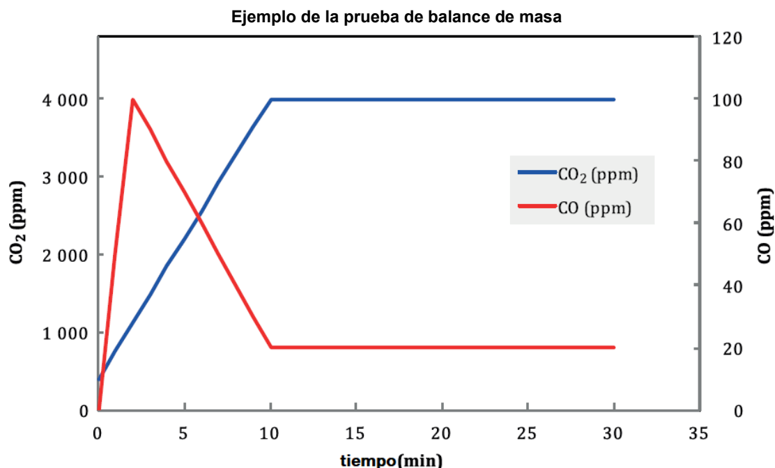
Figura C.3 - Concentraciones variables en el tiempo de CO 2 y CO en el tubo de muestra
