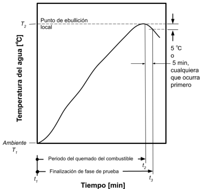
Figura 4 - Gráfico ilustrativo de la temperatura del agua contra el tiempo para cualquier fase de prueba cuando la temperatura del agua alcanza el punto de ebullición local al final del periodo de combustión del biocombustible
